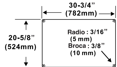
Borde Enrasado
