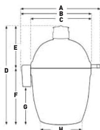
VISTA LATERALE
